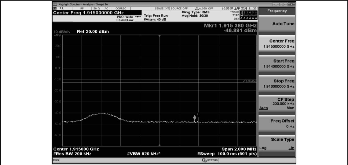
Band25-10MHz-QPSK-26640-50RB#0
