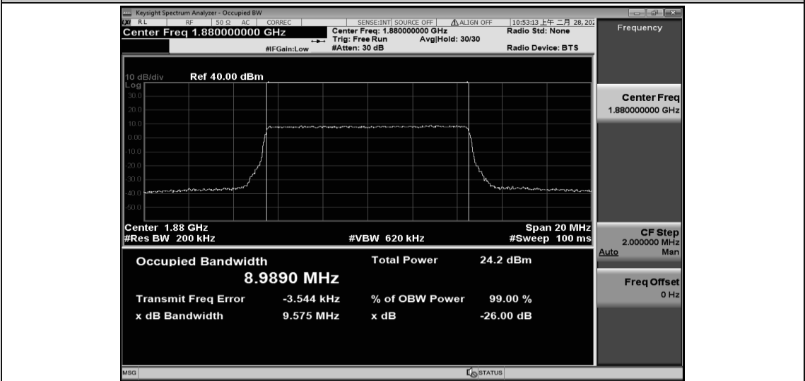
Band2-10MHz-QPSK-18800-50RB#0-8.9890
