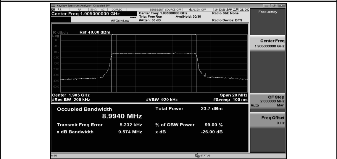
Band2-10MHz-QPSK-19050-50RB#0-8.9940
