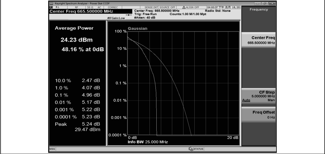
Band71-5MHz-QPSK-133147-25RB#0
