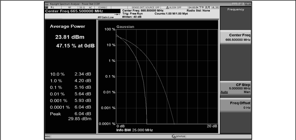
Band71-5MHz-QPSK-133297-1RB#0
