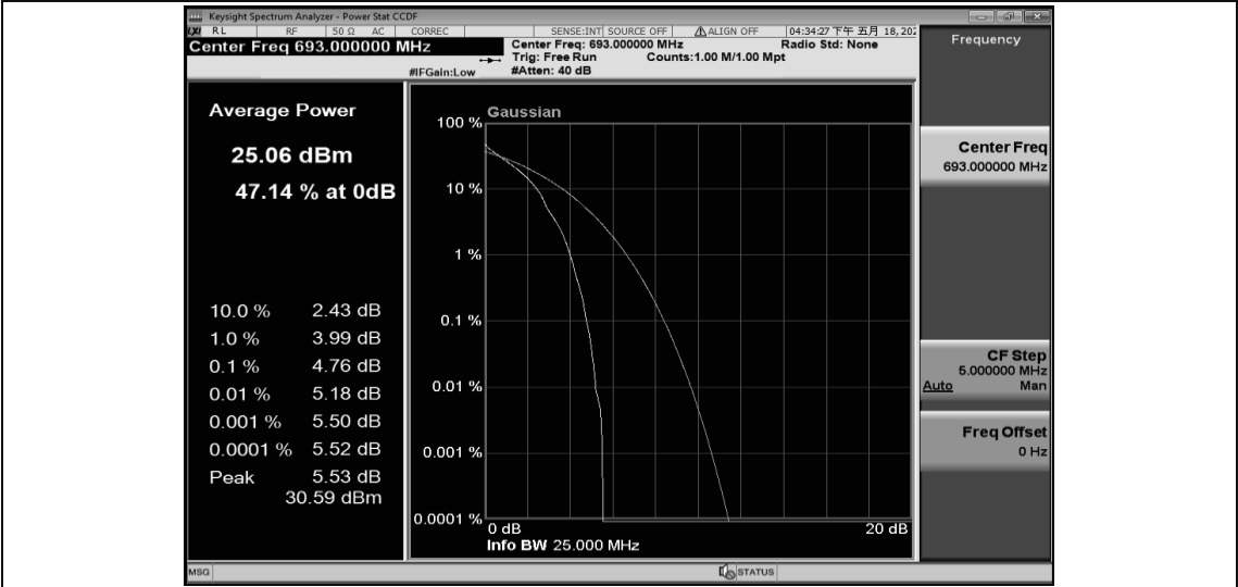
Band71-10MHz-QPSK-133422-50RB#0
