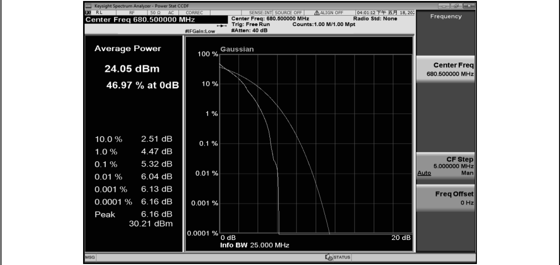
Band71-5MHz-QPSK-133297-25RB#0
