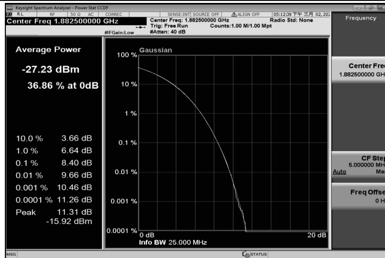
Band25-1.4MHz-QPSK-26365-6RB#0
