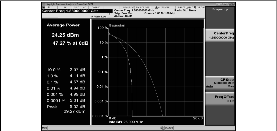
Band2-5MHz-QPSK-18900-25RB#0
