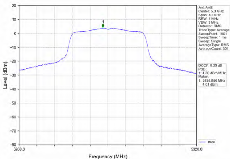
802.11a_MCH_5300MHz_Ant2_NTNV
