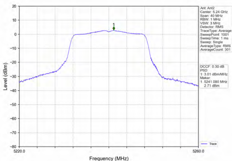
802.11a_HCH_5240MHz_Ant2_NTNV
