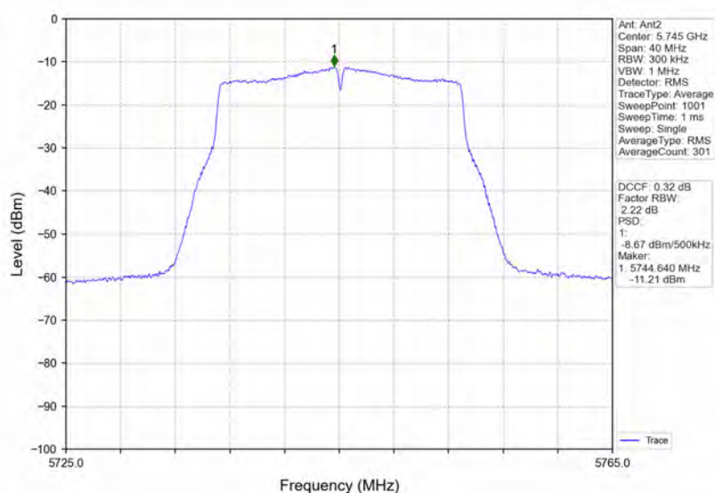
802.11n(HT20) LCH 5745MHz Ant2 NTVN
