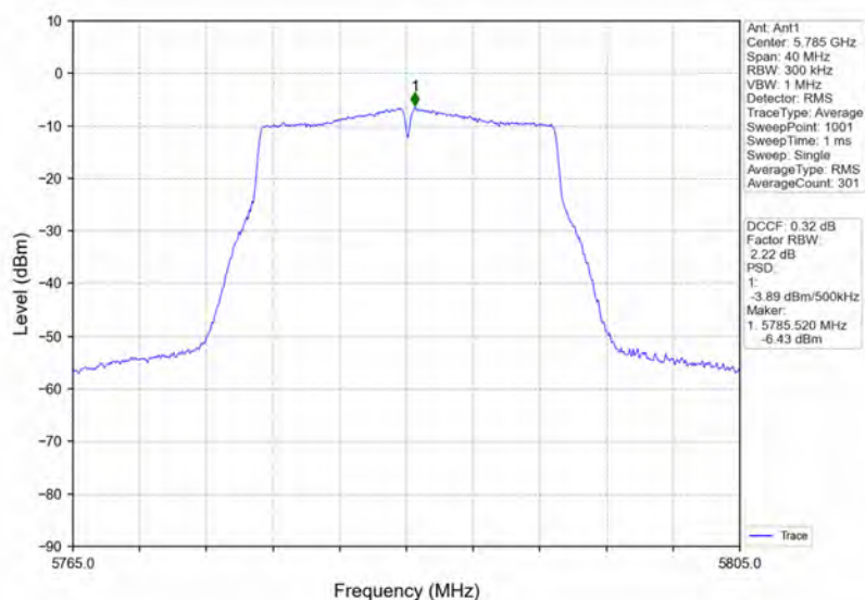
802.11n(HT20)_MCH_5785MHz_Ant1_NTNV
