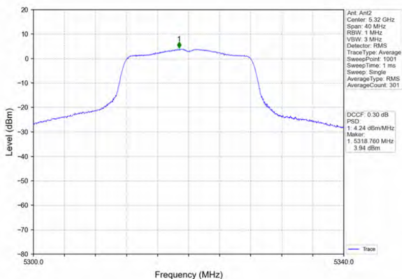
802.11a_HCH_5320MHz_Ant2_NTNV
