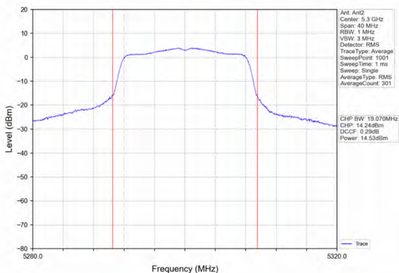
802.11a_MCH_5300MHz_Ant2_NTNV
