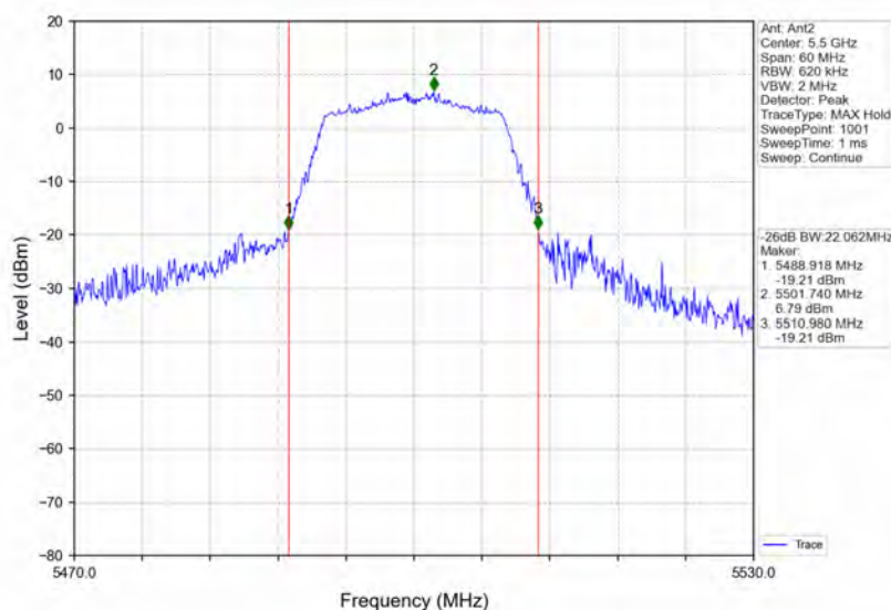
802.11a LCH_5500MHz_Ant2_NTNV
