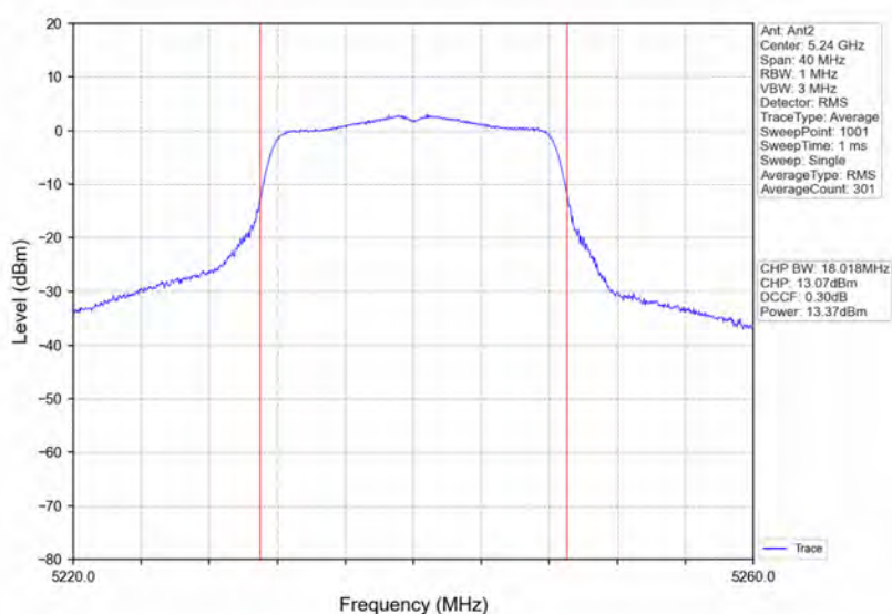
802.11a_HCH_5240MHz_Ant2_NTNV
