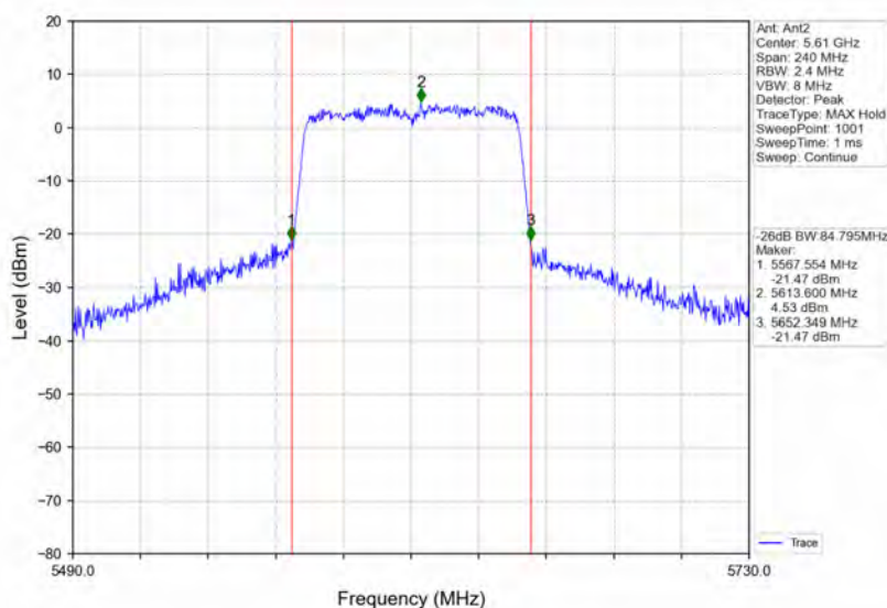
802.11ac(VHT80)_HCH_5610MHz_Ant2_NTNV
