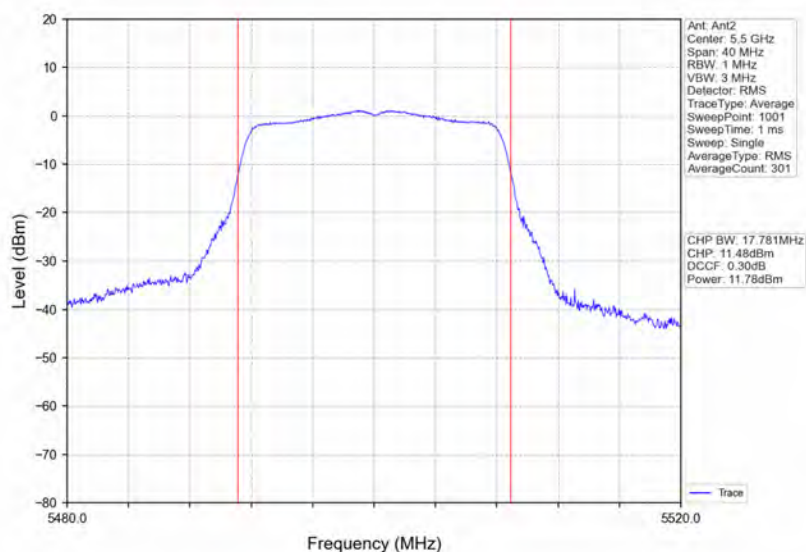
802.11a LCH_5500MHz_Ant2_NTNV
