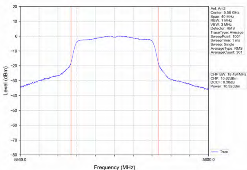
802.11a_MCH_5580MHz_Ant2_NTNV
