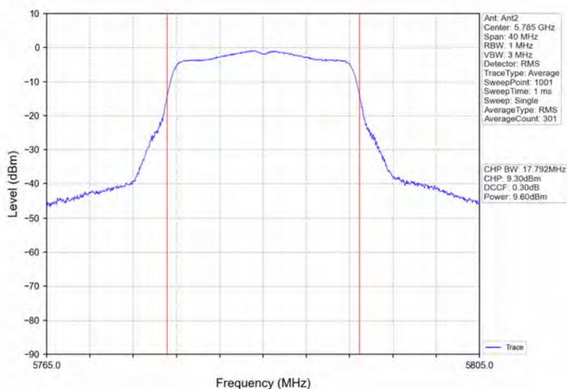
802.11a_MCH_5785MHz_Ant2_NTNV
