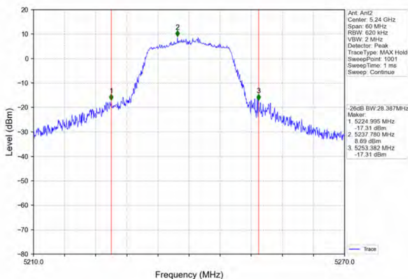
802.11a_HCH_5240MHz_Ant2_NTNV
