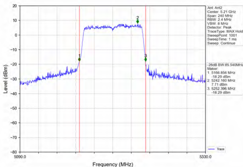
802.11ac(VHT80)_MCH_5210MHz_Ant2_NTNV
