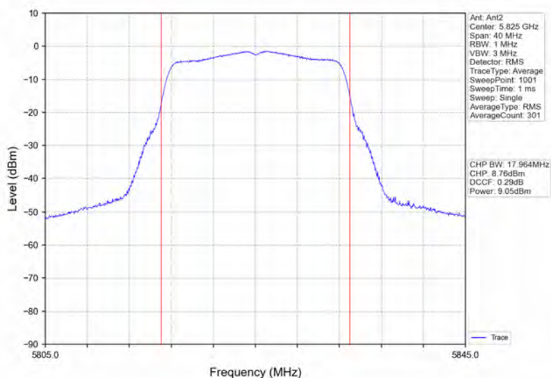
802.11a_HCH_5825MHz_Ant2_NTNV
