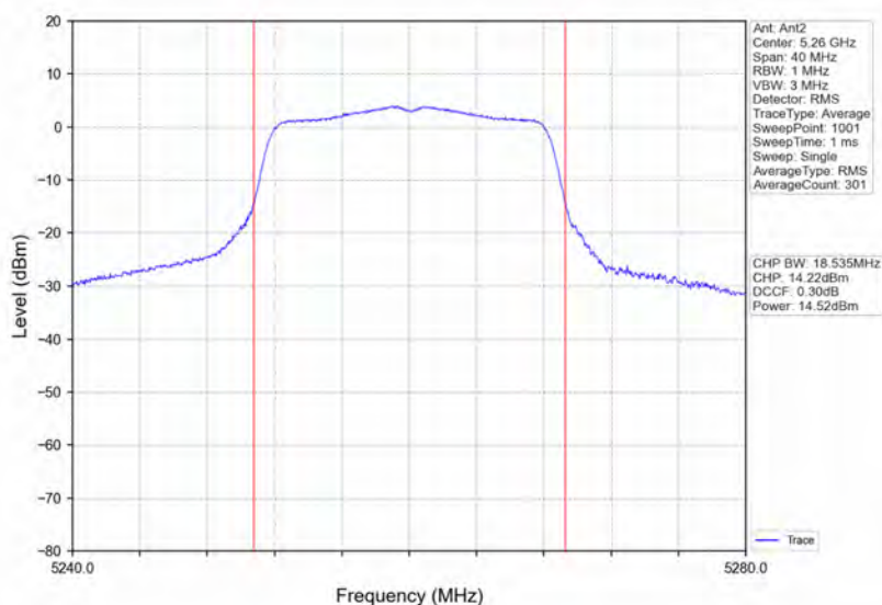
802.11a LCH_5260MHz_Ant2_NTNV
