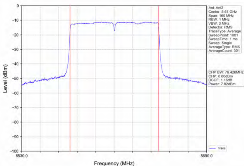
802.11ac(VHT80)_HCH_5610MHz_Ant2_NTNV
