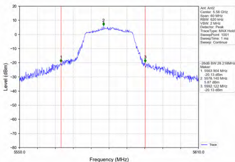
802.11a_MCH_5580MHz_Ant2_NTNV
