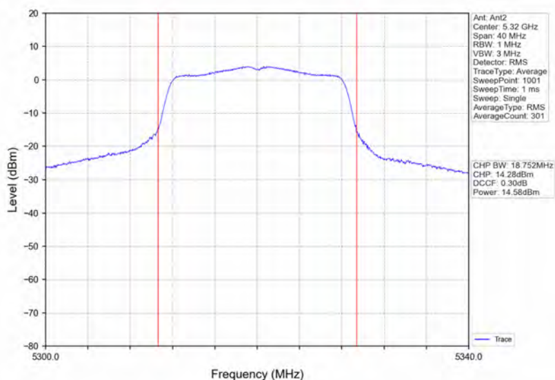
802.11a_HCH_5320MHz_Ant2_NTNV
