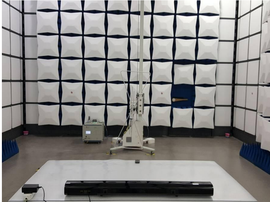
Above 1000MHz
