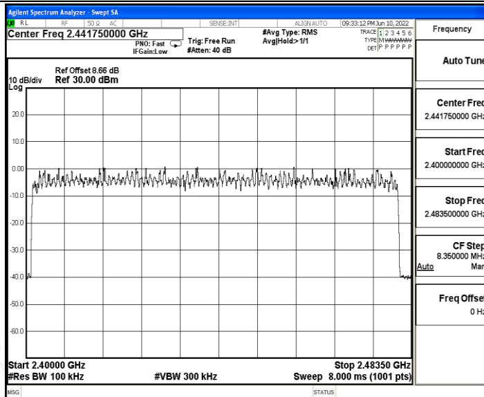
3DH5_Ant_Hop
