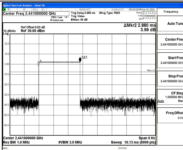
2DH5_Ant_Hop
