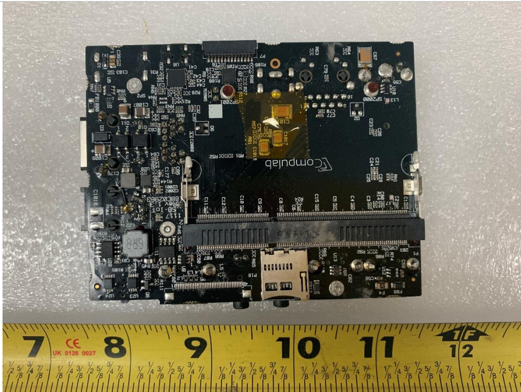
EUT PCBA2 - Bottom
