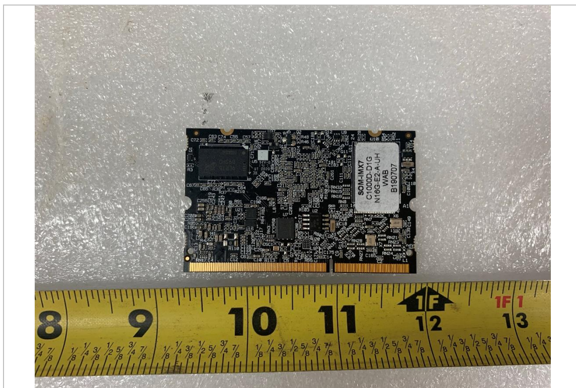
EUT PCBA4 - Bottom
