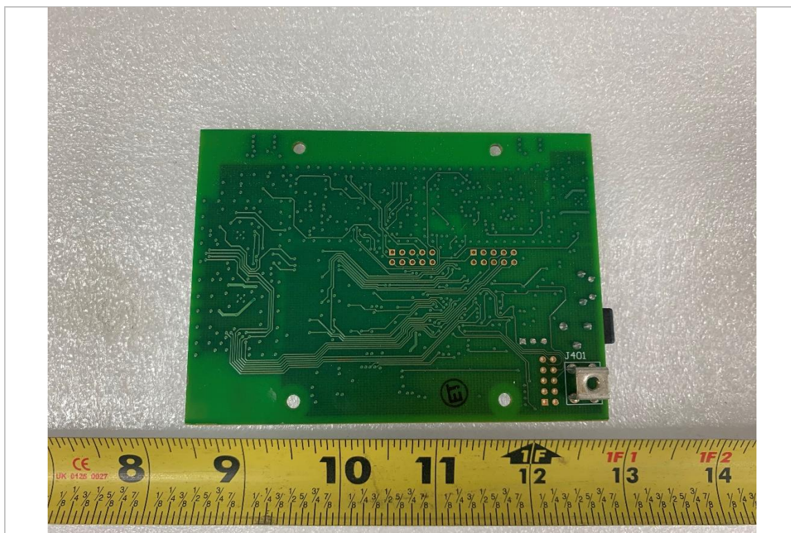
EUT PCBA5 - Bottom
