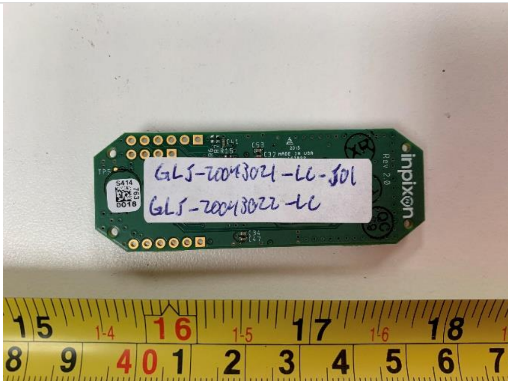
UWB Module – Bottom
