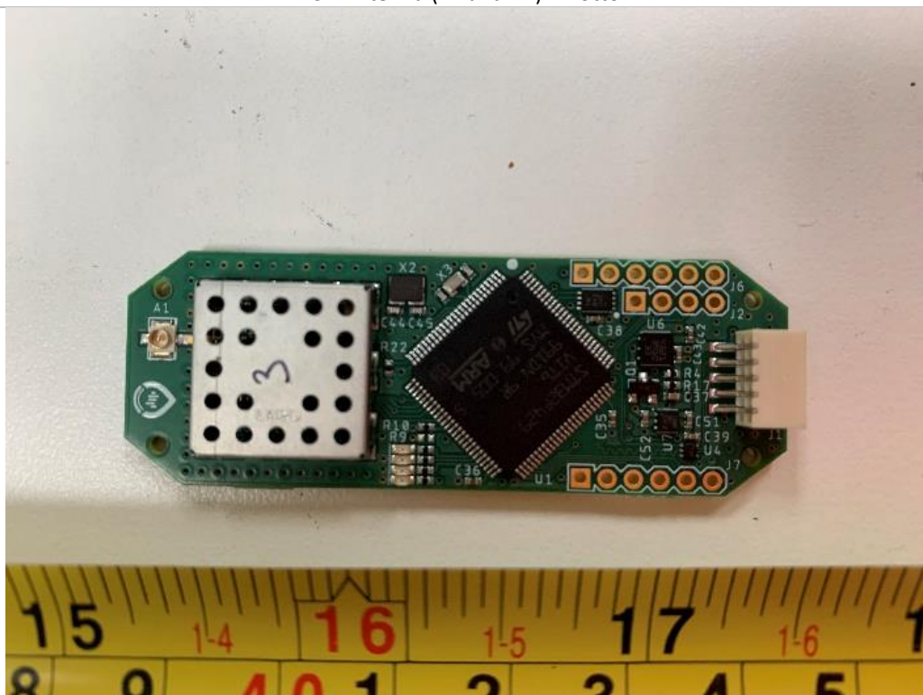
UWB Module - Top
