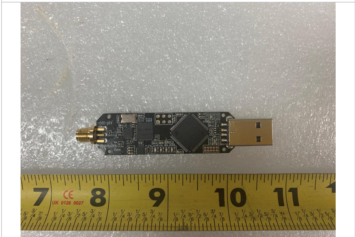
EUT PCBA1 - Top
