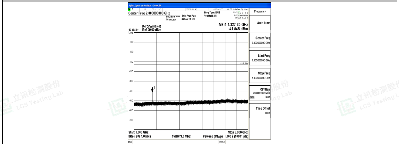
Band71_10MHz_QPSK_133172_1RB#0_1000~3000_1000~3000
