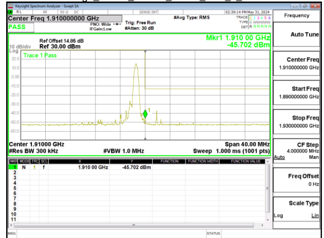
Band Edge_Band2_20MHz_QPSK_RB6_0_CH18700
