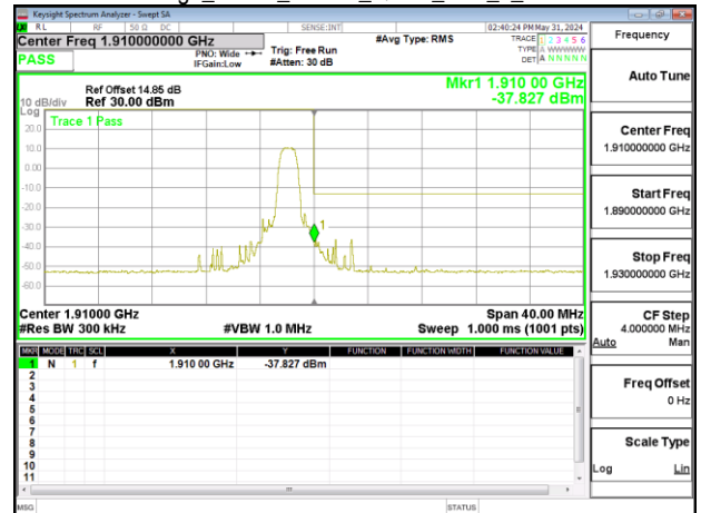
Band Edge_Band2_20MHz_QPSK_RB6_0_CH19100
