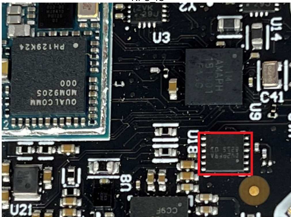
NFC IC
