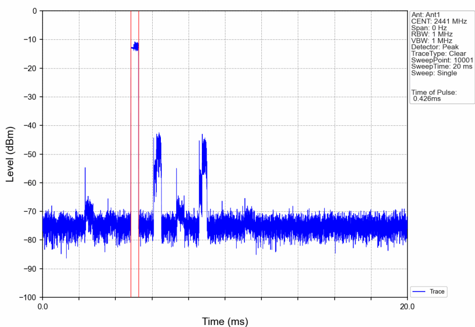
8-DPSK_3DH1_HOPP_Ant1_NTNV
