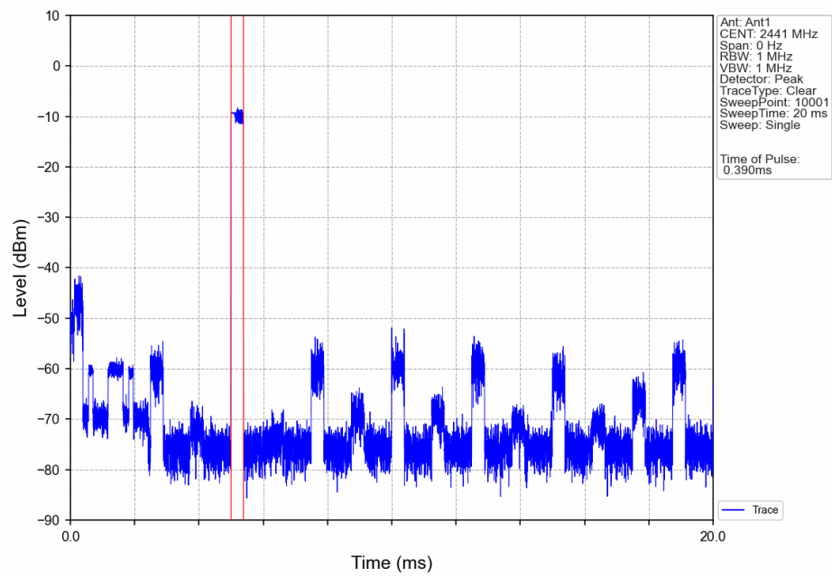
8-DPSK_3DH1_HOPP_Ant1_NTNV
