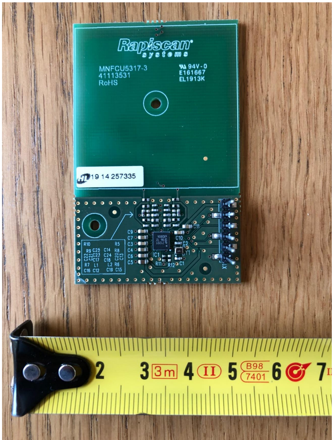
NFC module component side
