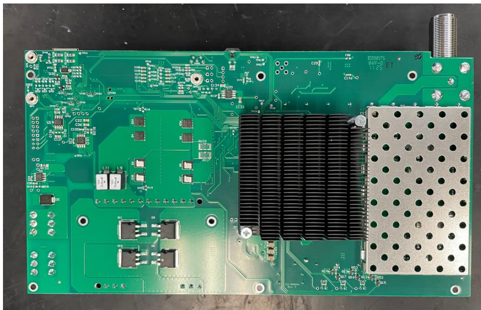
PCA Bottom View
