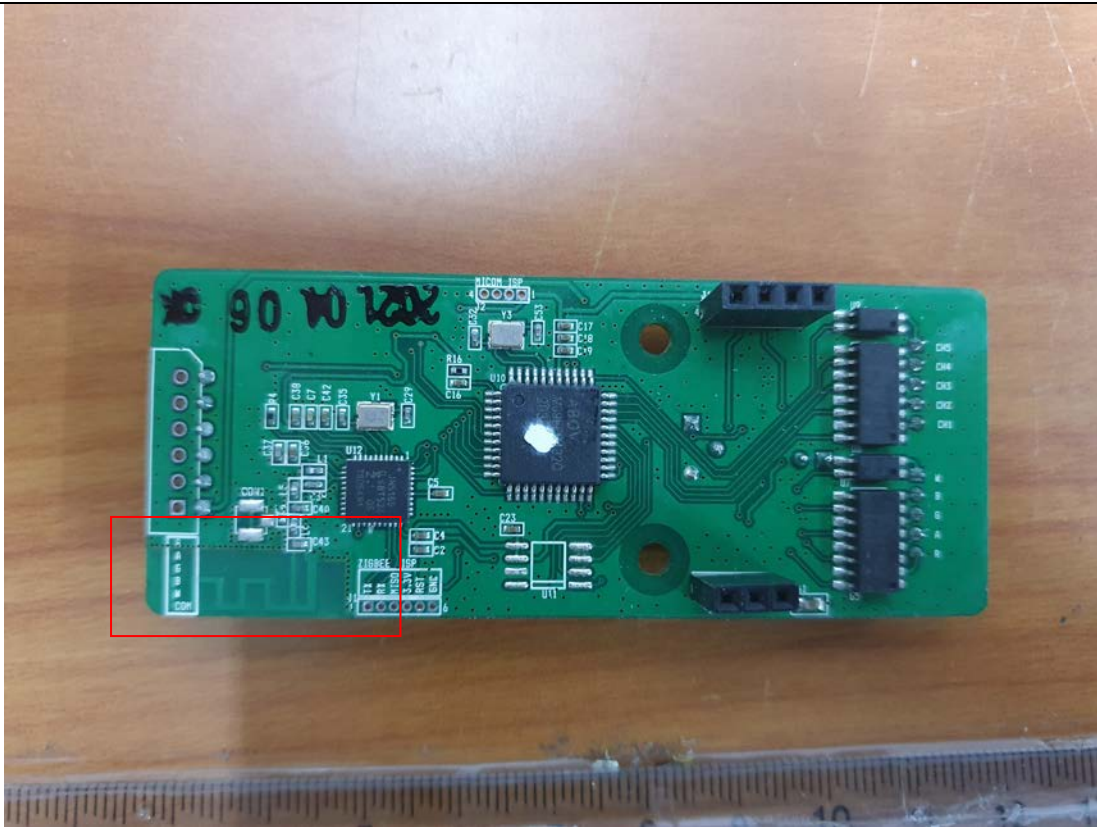
ANTENNA(2.4 GHz)
