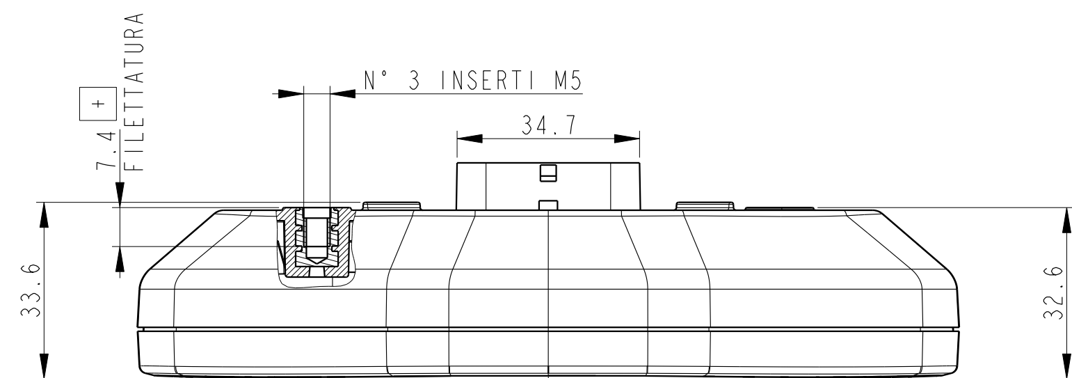
SEZIONE B-B
