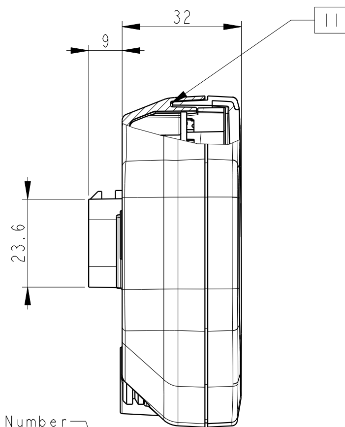
SEZIONE E-E
