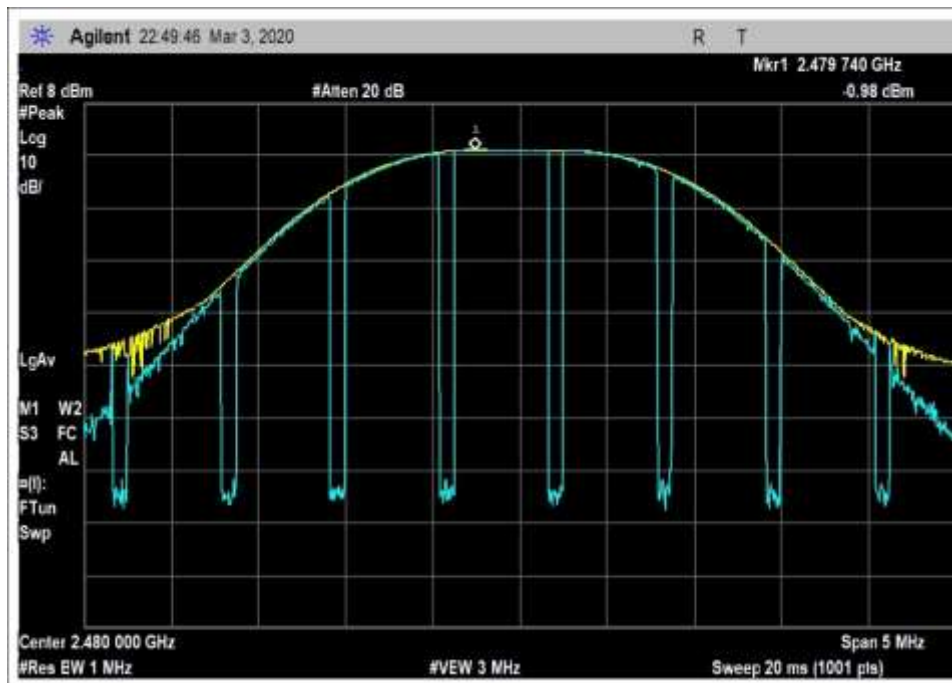
2480 BLE Vnom
