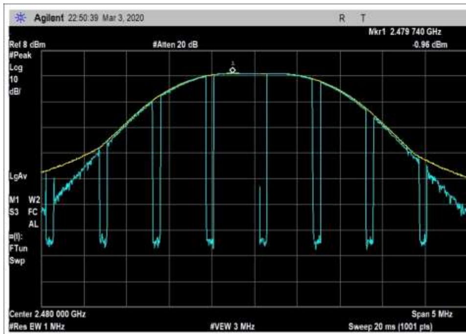
2480 BLE Vmax
