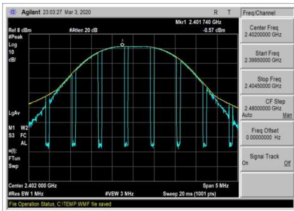
2402 BLE Vnom
