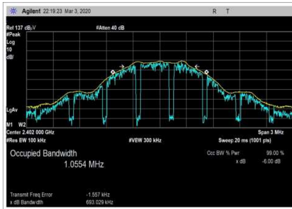
2402 BLE
