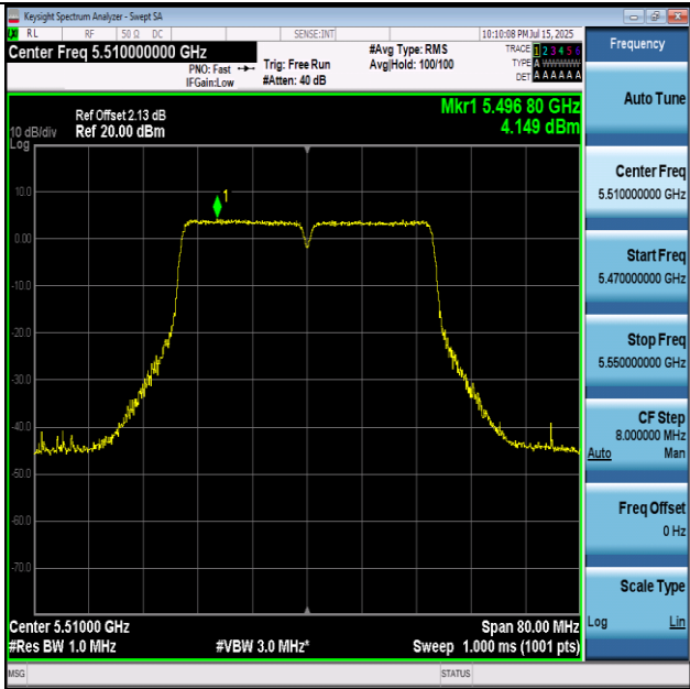
11N40-5510-PASS
