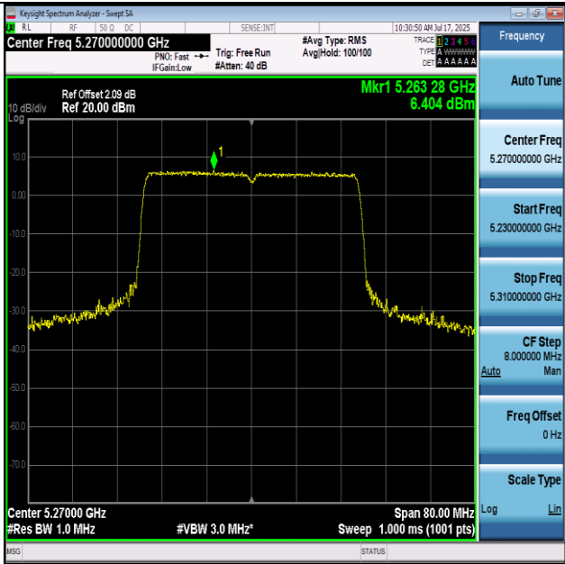
11AX40-5270-PASS
