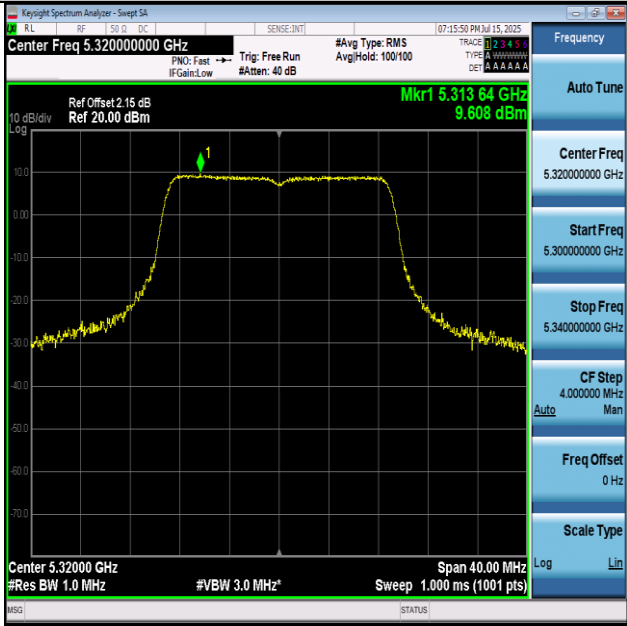
11N20-5320-PASS
