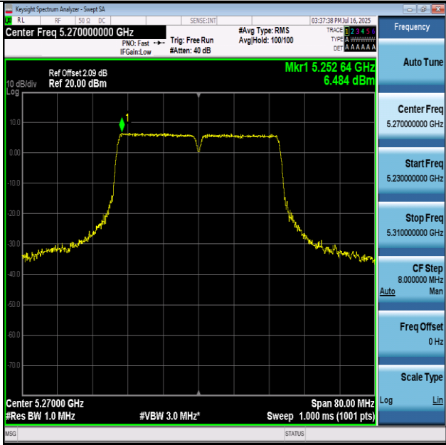
11AC40-5270-PASS
