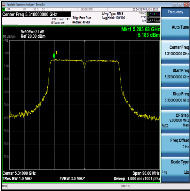
11AC40-5310-PASS
