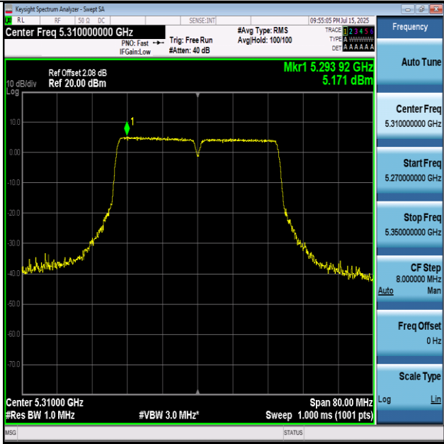
11N40-5310-PASS
