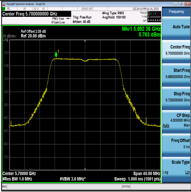
11AC20-5700-PASS
