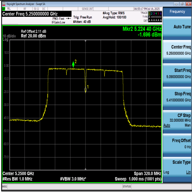
11AC160-5250_UNII-1-PASS
