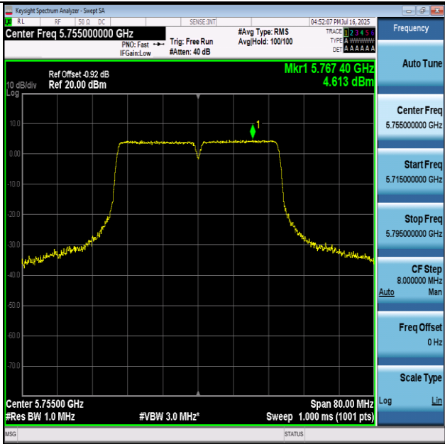
11AC40-5755-PASS
