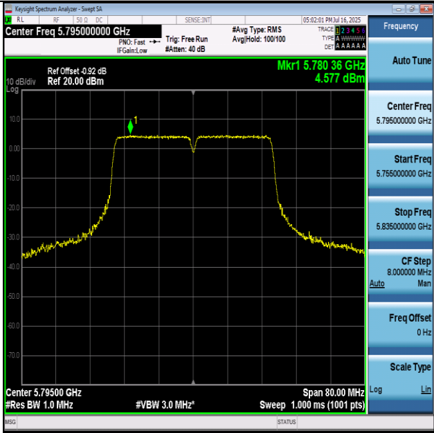
11AC40-5795-PASS
