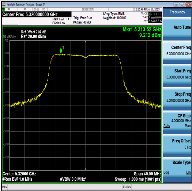
11AC20-5320-PASS
