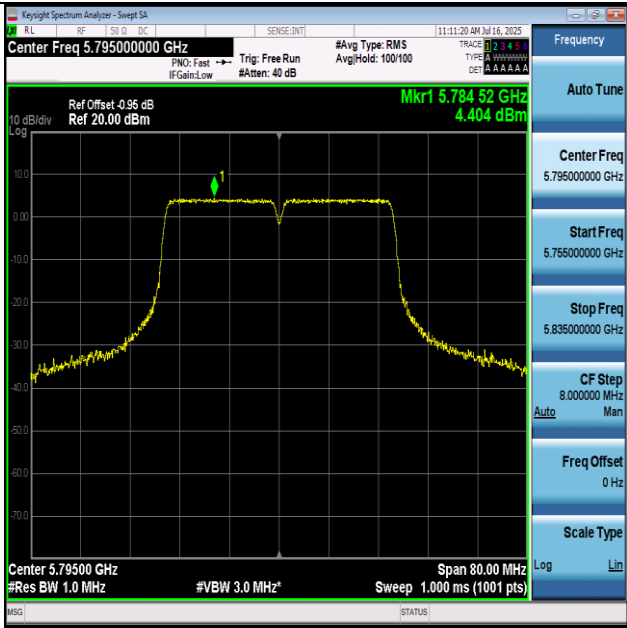
11N40-5795-PASS
