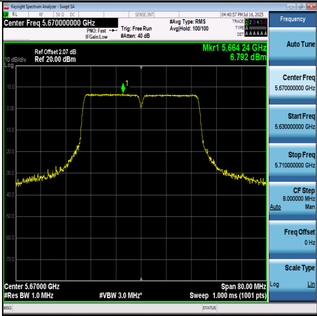
11AC40-5670-PASS
