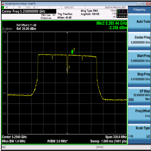
11AC160-5250_UNII-2A-PASS
