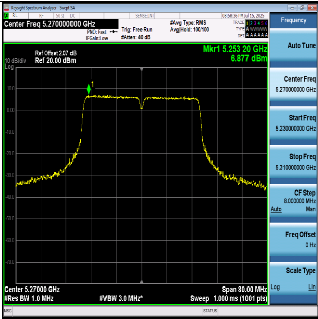
11N40-5270-PASS
