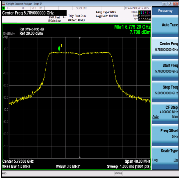
11AC20-5785-PASS
