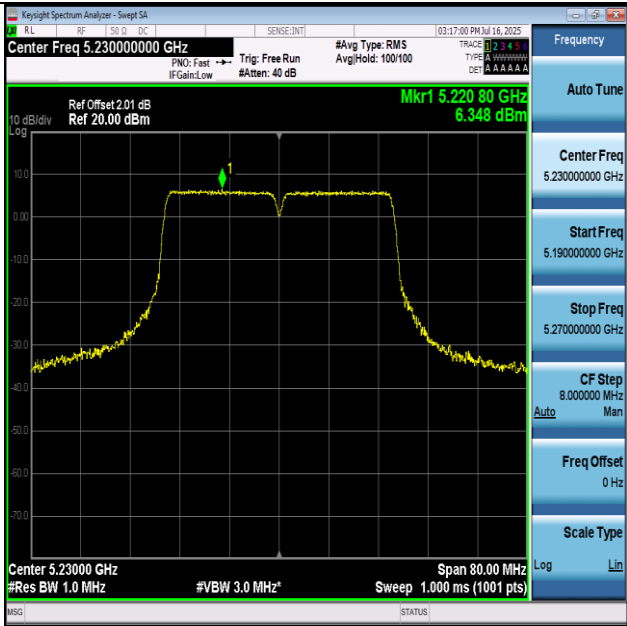
11AC40-5230-PASS
