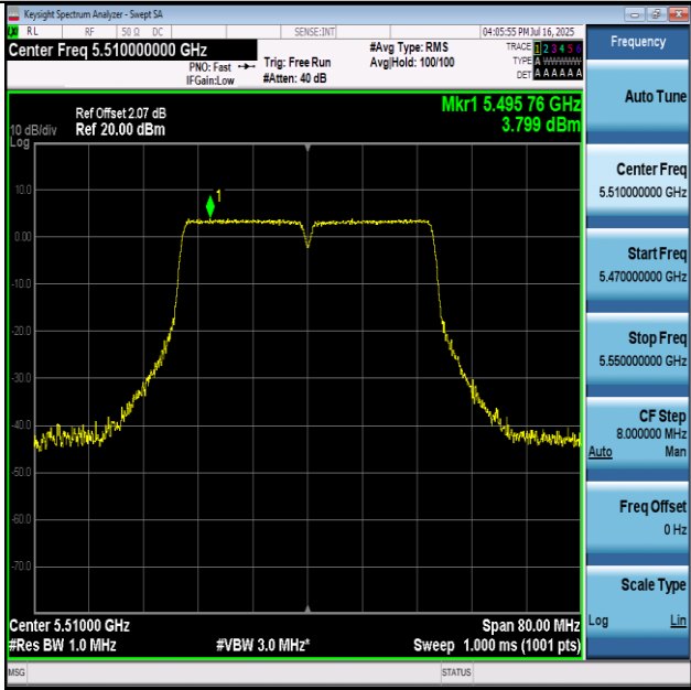
11AC40-5510-PASS
