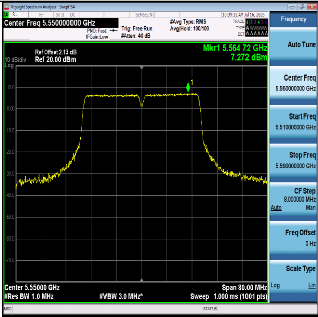
11N40-5550-PASS
