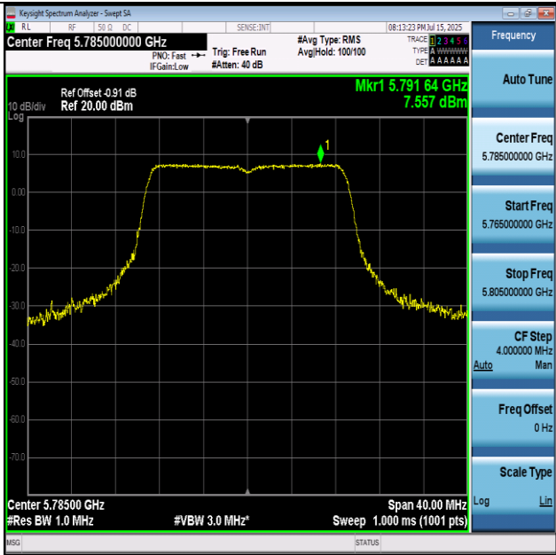
11N20-5785-PASS
