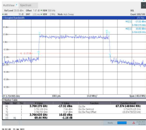
1-N78-3700-3800--30-70-L-6-CP-QPSK-Out_Full-1 89@0-Ant1-67.574-69.440-≤70-PASS
