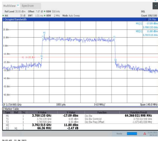
1-N78-3700-3800--30-70-L-4-DFT-64QAM-Out_Ful I-180@0-Ant1-64.366-66.360-≤70-PASS
