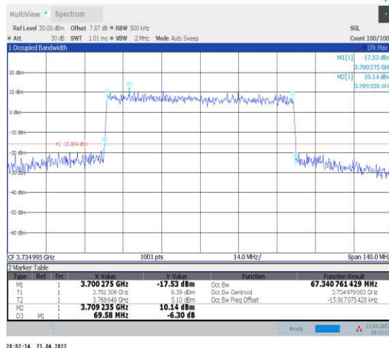
1-N78-3700-3800--30-70-L-7-CP-16QAM-Out_Full -189@0-Ant1-67.341-69.580-≤70-PASS
