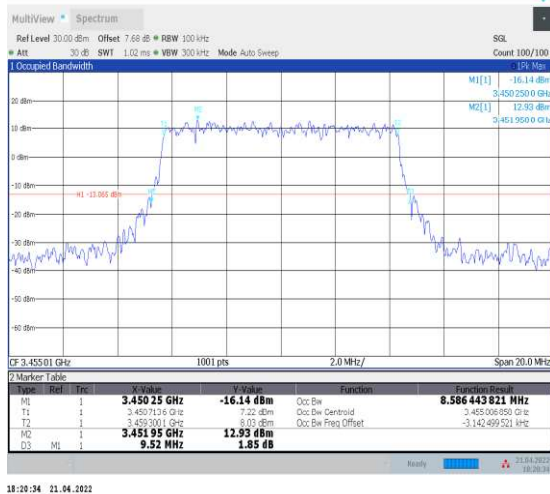
1-N78-3450-3550--30-10-L-3-DFT-16QAM-Out_Ful I-24@0-Ant1-8.586-9.520-≤10-PASS
