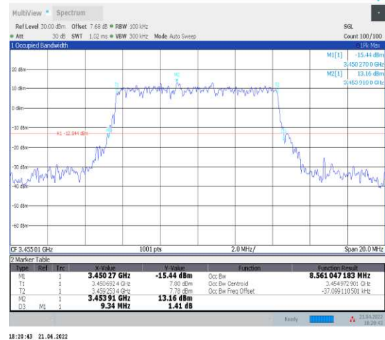
1-N78-3450-3550--30-10-L-4-DFT-64QAM-Out_Fu II-24@0-Ant1-8.561-9.340-≤10-PASS
