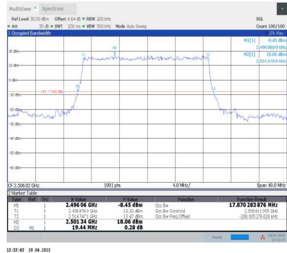
1-N41--30-20-L-2-DFT-PI2BPSK-Outer_Full-50@0-A nt1-17.87-19.440-≤20-PASS
