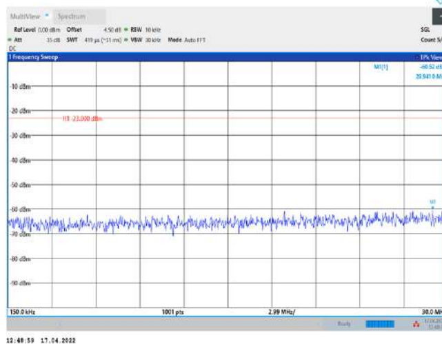
Band71-20MHz-QPSK-133222-1RB#0-Range2:0.15~30MHz
