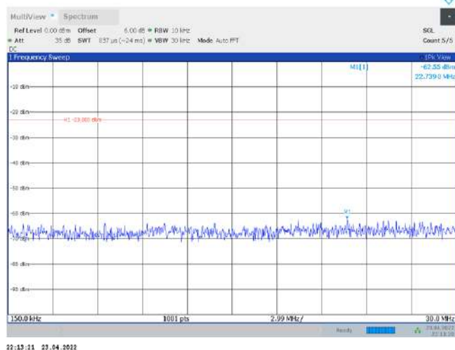
Band43-20MHz-QPSK-44690-1RB#0-Range2:0.15~30MHz
