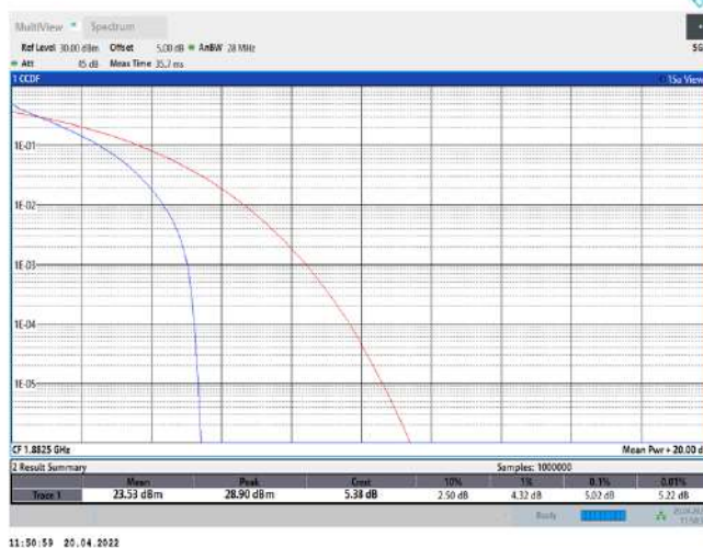
Band25-20MHz-QPSK-26365-100RB#0
