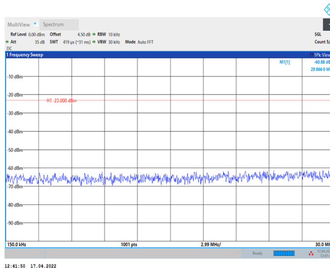
Band13-10MHz-QPSK-23230-1RB#0-Range2:0.15~30MHz
