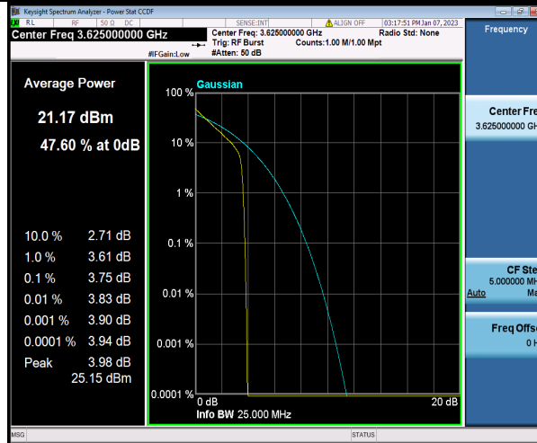
N48-20MHz-QPSK-641666-50RB#0
