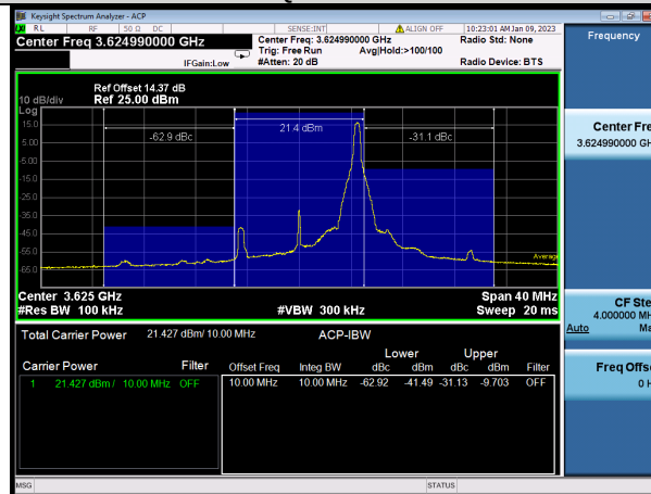
N48-10MHz-QPSK-641666-25RB#0
