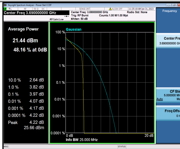
N48-20MHz-QPSK-646000-50RB#0
