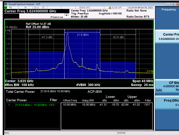
N48-10MHz-QPSK-641666-1RB#24
