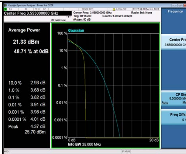
Band48-10MHz-QPSK-55290-50RB#0
