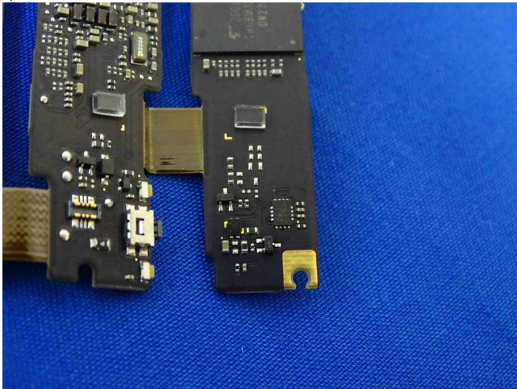
(40) EUT Photo
