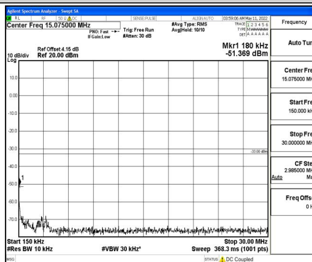
Band2-20MHz-16QAM-18700-1RB#0-Range3:30~1000MHz
