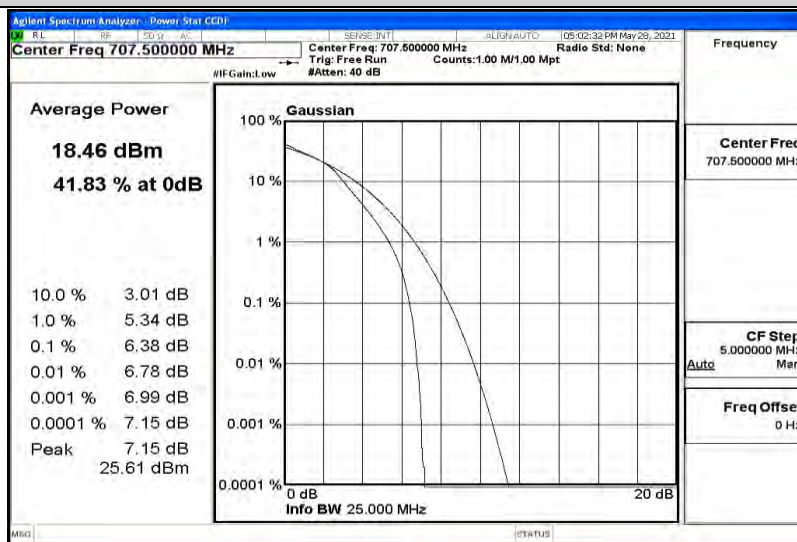
Band12-3MHz-QPSK-23165-15RB#0
