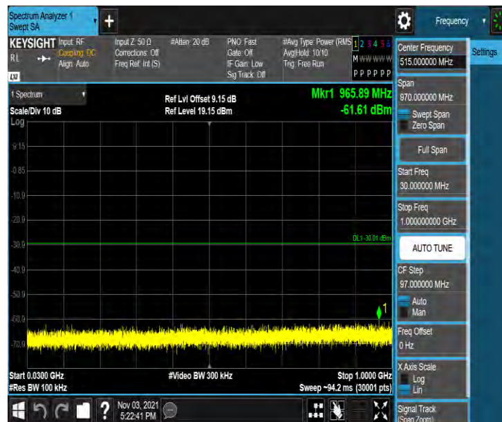
11G_Ant1_2412_30~1000
