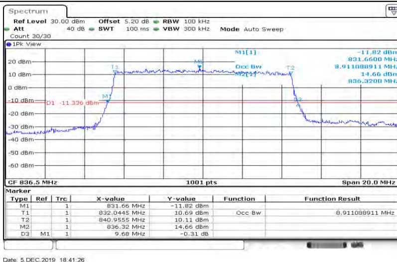
Band5-10MHz-QPSK-20600-50RB#0-8.911
