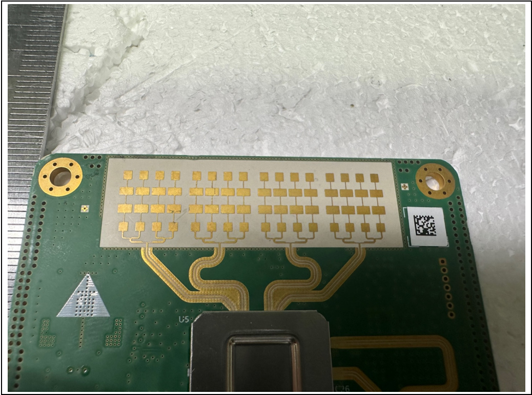
<RX Antenna>
