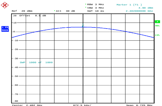
\pi/4 -DQPSK_Low 4.90dBm
