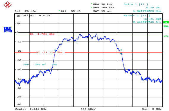
\pi/4 -DQPSK_Middle 1.348MHz
