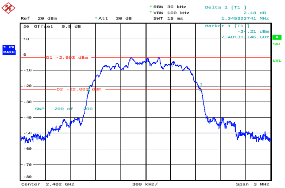
\pi/4 -DQPSK_Low 1.345MHz
