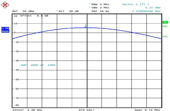
\pi/4 -DQPSK_High 5.11dBm
