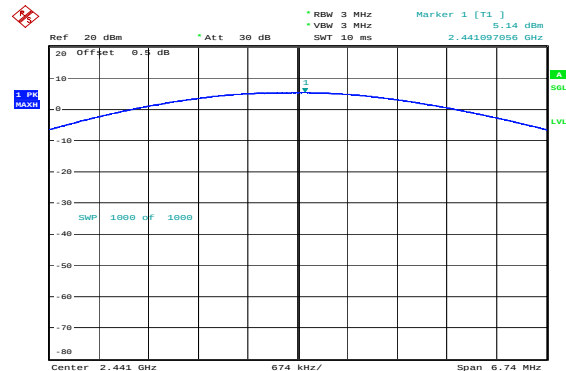
\pi/4 -DQPSK_Middle 5.14dBm
