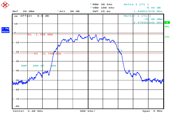
\pi/4 -DQPSK_High 1.341MHz
