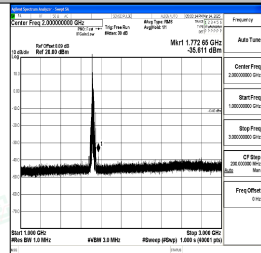
Band66_20MHz_QPSK_132072_1RB#0_1000~ 3000_1000~3000
