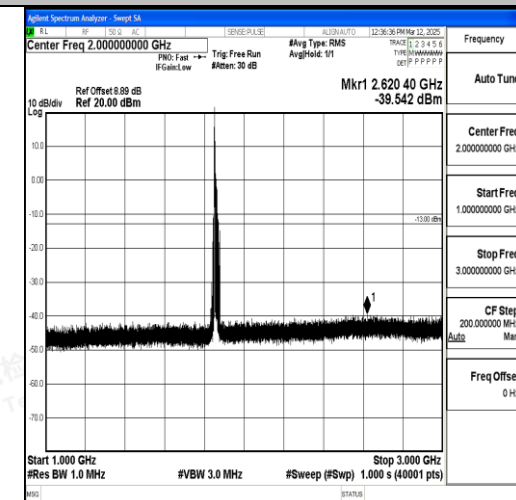
Band2_15MHz_QPSK_18675_1RB#0_1000~300 0_1000~3000
