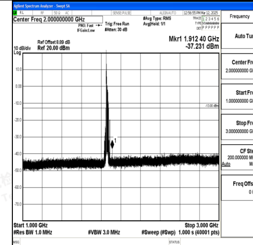
Band2_20MHz_QPSK_18700_1RB#0_1000~300 0_1000~3000
