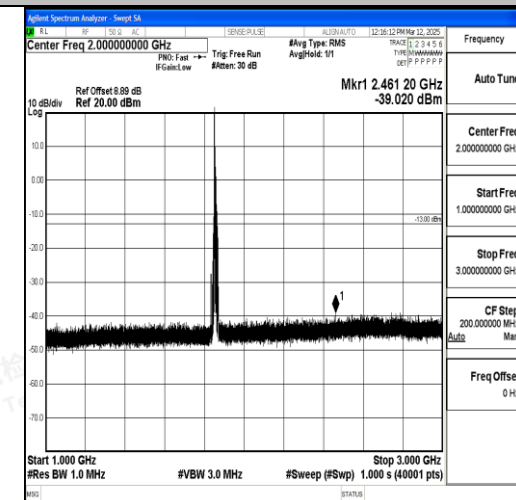
Band2_10MHz_QPSK_18650_1RB#0_1000~300 0_1000~3000
