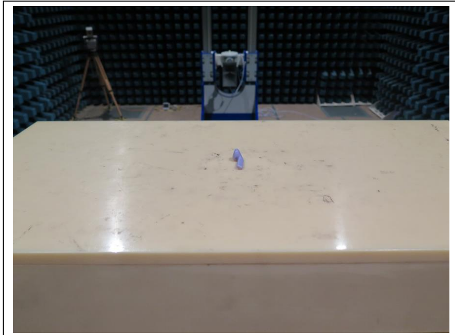
EUT Position
