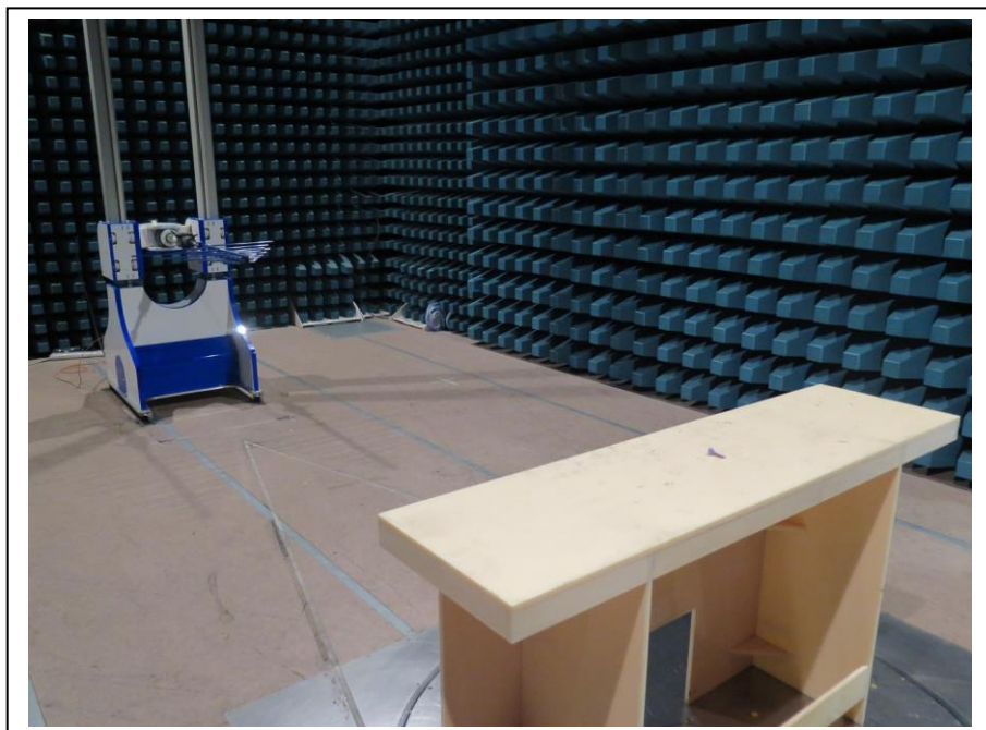
200MHz – 1GHz
