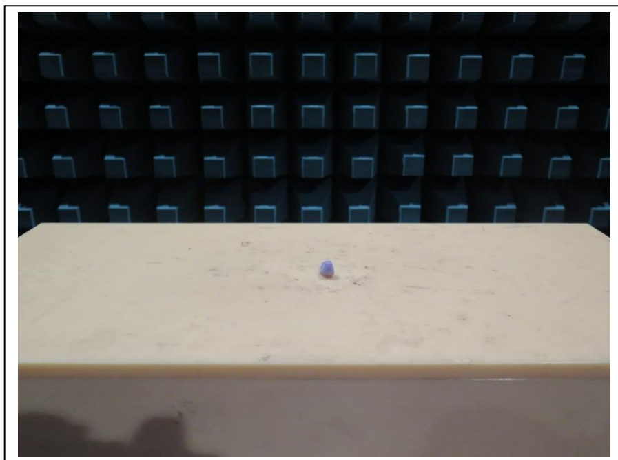
EUT position
