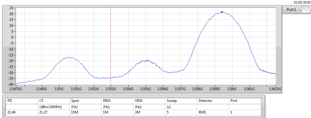
Band 48_LTE_10MHz_Nss1,QPSK_1TX 3555MHz_QPSK_RB 1,#RB H
