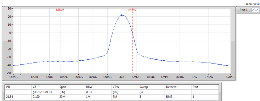
Band 48_LTE_20MHz_Nss1,QPSK_1TX 3690MHz_QPSK_RB 1,#RB M
