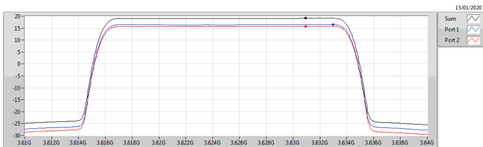
Band 48_LTE_20MHz_Nss1,QPSK_2TX 3625MHz_QPSK_RB 100,#RB 0
