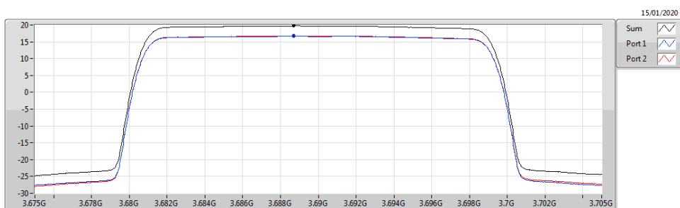
Band 48_LTE_20MHz_Nss1,QPSK_2TX 3690MHz_QPSK_RB 100,#RB 0
