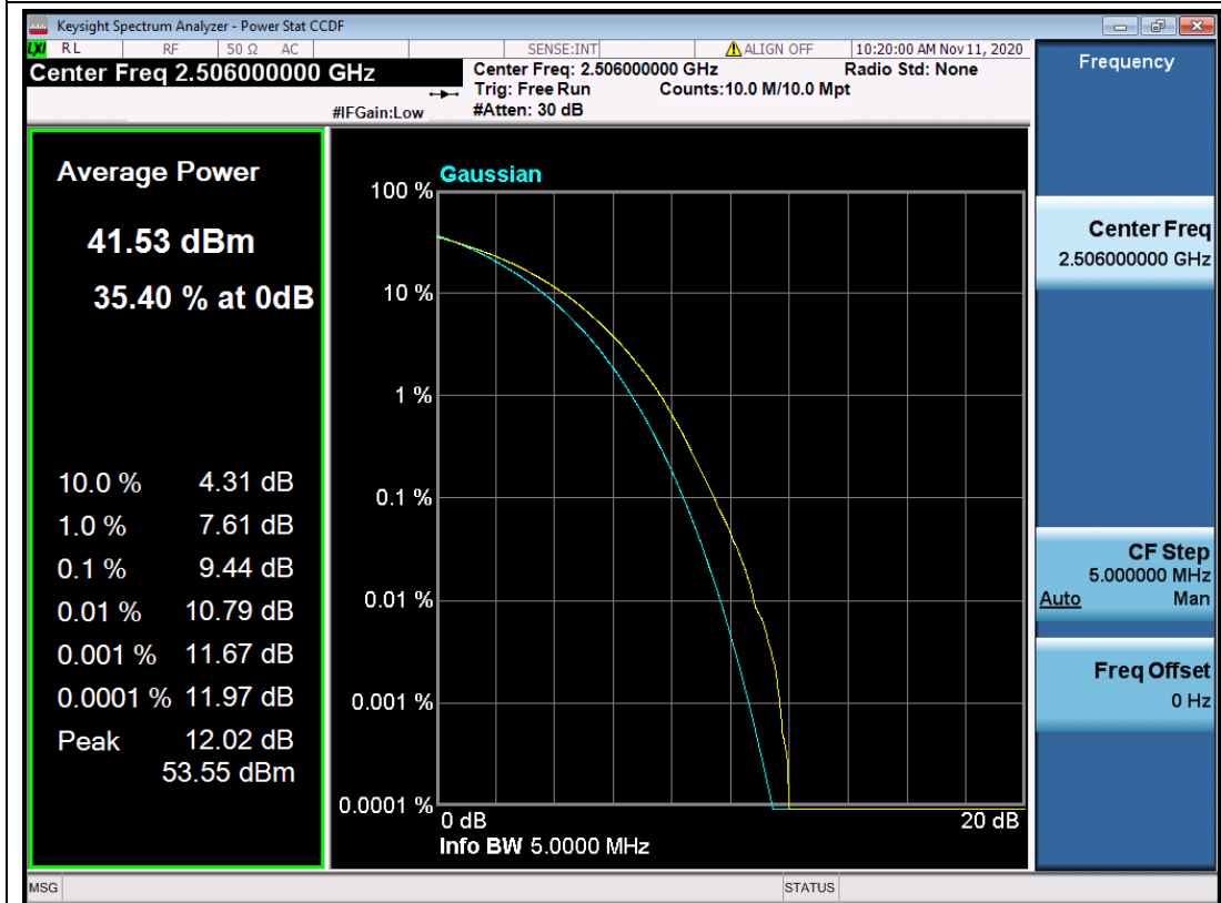
B41-20-PAPR-Q64-L.png
