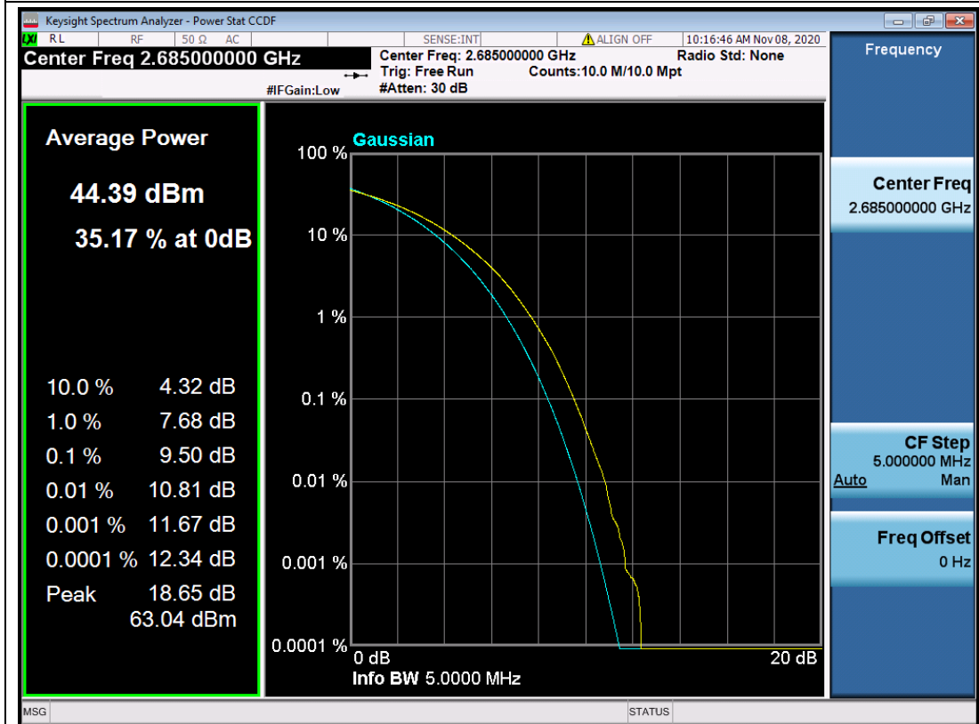
B41-10-PAPR-QPSK-H.png
