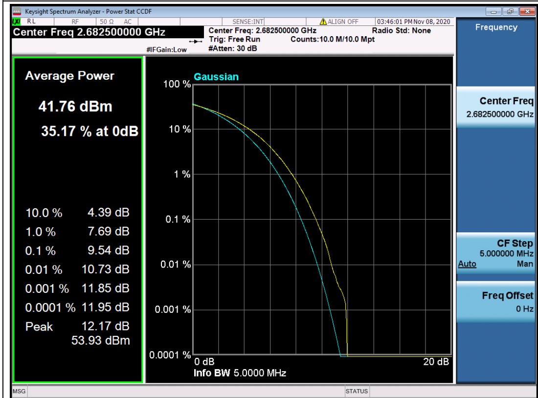
B41-15-PAPR-Q64-H.png
