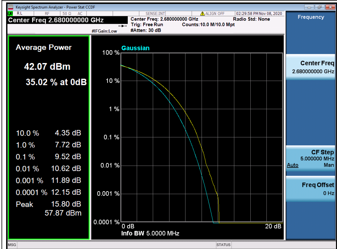
B41-20-PAPR-QPSK-H.png
