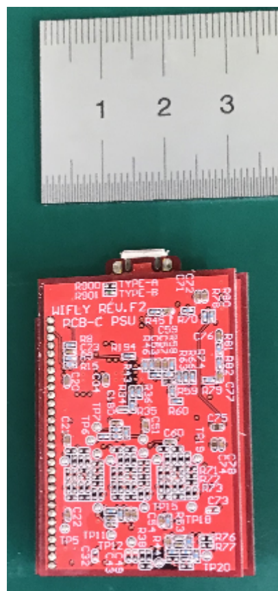
PCB_4: Bottom
