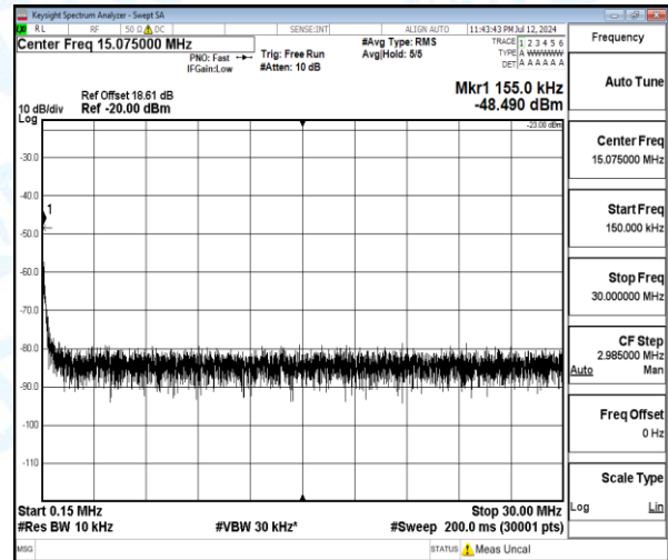
Band12-3MHz-QPSK-23095-1-0-Low-0.15-30-0.15--48.49-25.49--23-PASS
