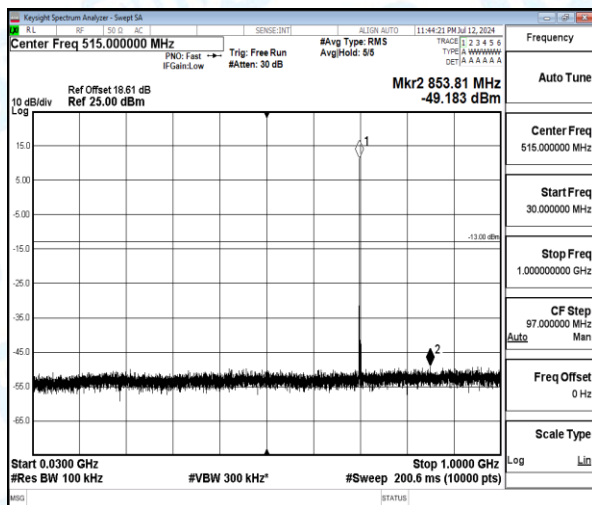
Band12-3MHz-16QAM-23095-1-0-Low-30-1000-853.81--49.18-36.18--13-PASS
