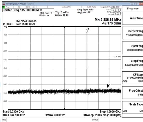
Band12-1.4MHz-QPSK-23095-1-0-Low-30-1000-886.69--49.17-36.17--13-PASS
