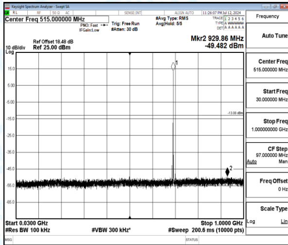
Band12-1.4MHz-QPSK-23017-1-0-Low-30-1000-929.86--49.48-36.48--13-PASS
