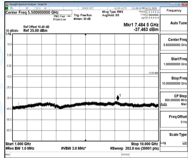
Band12-1.4MHz-QPSK-23017-1-0-Low-1000-10000-7484.5--37.46-24.46--13-PASS
