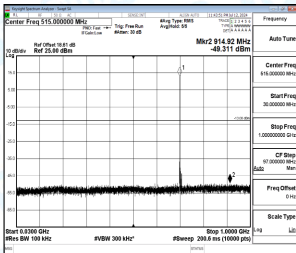
Band12-3MHz-QPSK-23095-1-0-Low-30-1000-914.92--49.31-36.31--13-PASS
