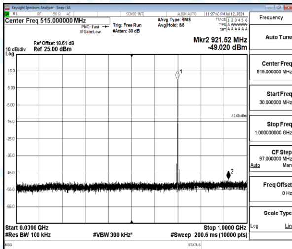
Band12-1.4MHz-16QAM-23095-1-0-Low-30-1000-921.52--49.02-36.02--13-PASS
