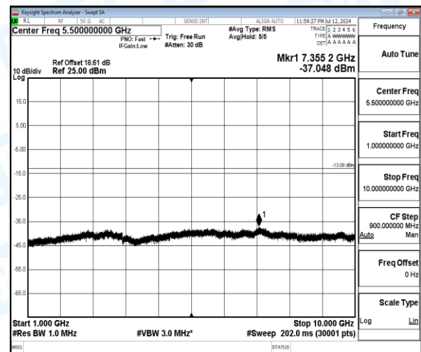
Band12-5MHz-QPSK-23095-1-0-Low-1000-10000-7355.2--37.05-24.05--13-PASS
