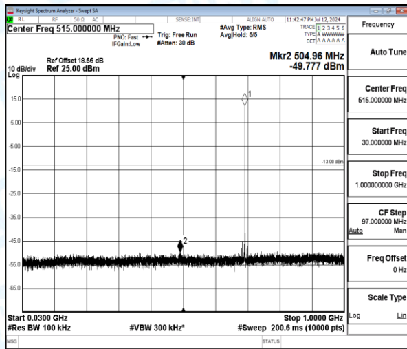
Band12-3MHz-QPSK-23025-1-0-Low-30-1000-504.96--49.78-36.78--13-PASS
