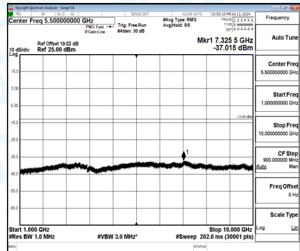
Band5-5MHz-16QAM-20425-1-0-Low-1000-10000-7325.5--37.02-24.02--13-PASS
