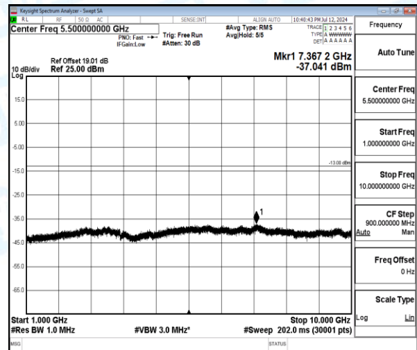
Band5-3MHz-QPSK-20415-1-0-Low-1000-10000-7367.2--37.04-24.04--13-PASS
