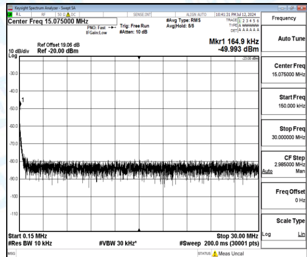
Band5-3MHz-QPSK-20525-1-0-Low-0.15-30-0.16--49.99-26.99--23-PASS
