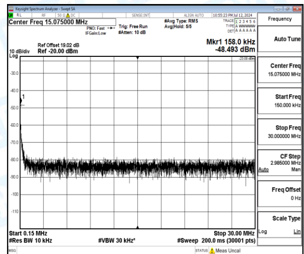
Band5-5MHz-QPSK-20425-1-0-Low-0.15-30-0.16--48.49-25.49--23-PASS
