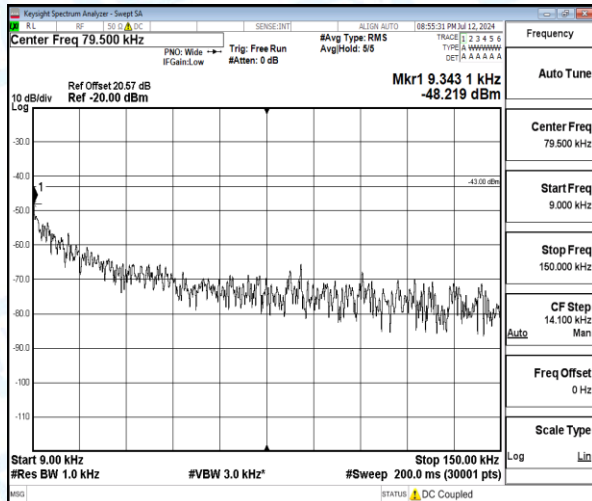
Band4-5MHz-QPSK-19975-1-0-Low-0.009-0.15-0.01--48.22-5.22--43-PASS
