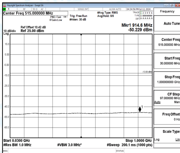
Band4-3MHz-16QAM-19965-1-0-Low-30-1000-914.55--50.23-37.23--13-PASS
