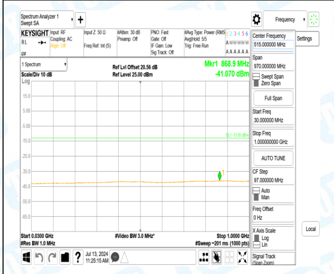
Band4-3MHz-QPSK-20175-1-0-Low-30-1000-868.92--41.07-28.07--13-PASS
