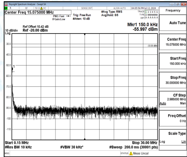
Band4-1.4MHz-QPSK-19957-1-0-Low-0.15-30-0.15--56-23--33-PASS
