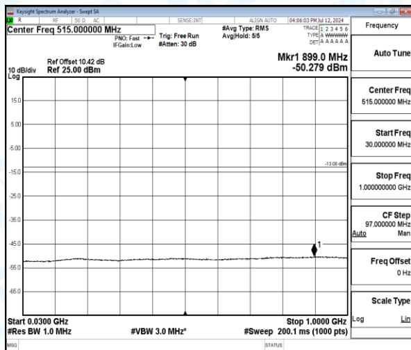
Band4-1.4MHz-QPSK-19957-1-0-Low-30-1000-899.02--50.28-37.28--13-PASS
