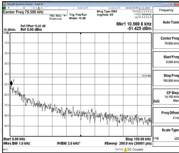
Band4-1.4MHz-QPSK-19957-1-0-Low-0.009-0.15-0.01-51.43-8.43--43-PASS
