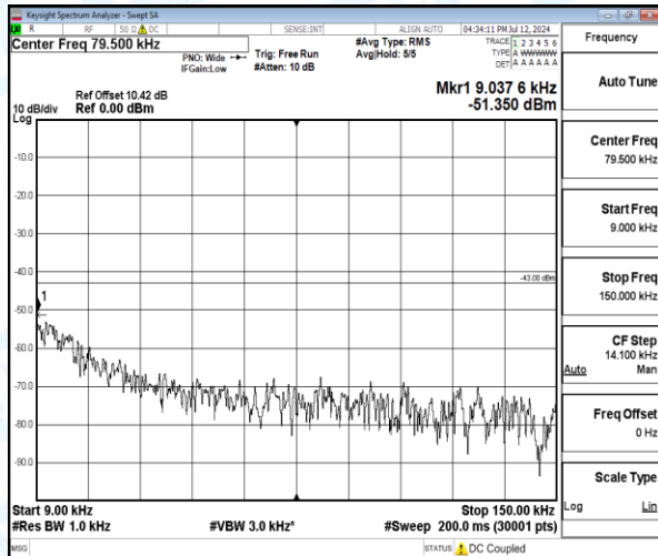
Band4-3MHz-QPSK-19965-1-0-Low-0.009-0.15-0.01--51.35-8.35--43-PASS
