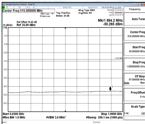
Band4-3MHz-QPSK-19965-1-0-Low-30-1000-894.16--50.27-37.27--13-PASS
