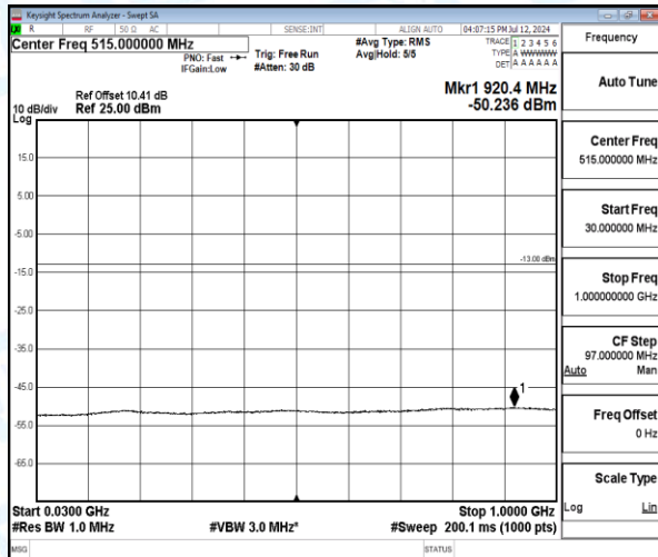
Band4-1.4MHz-QPSK-20175-1-0-Low-30-1000-920.38--50.24-37.24--13-PASS
