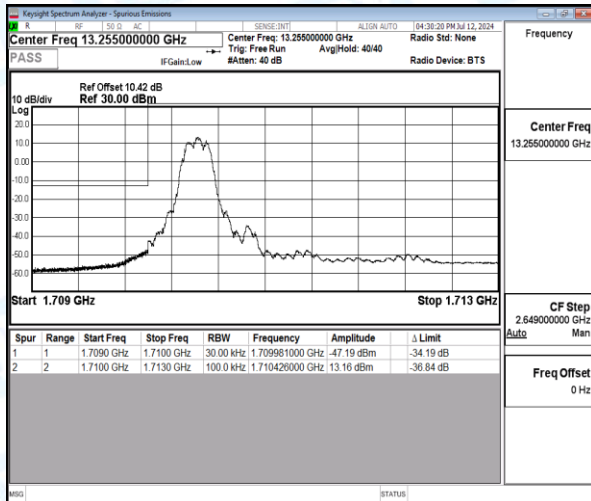
Band4-3MHz-16QAM-19965-1-0-Low-1709.98--47.19-34.19-PASS
