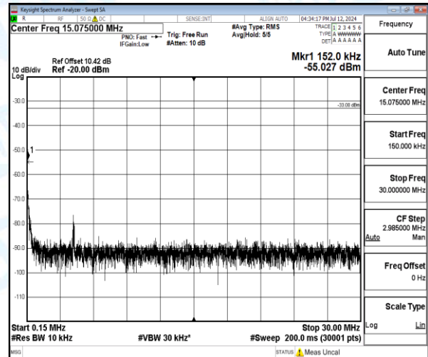
Band4-3MHz-QPSK-19965-1-0-Low-0.15-30-0.15--55.03-22.03--33-PASS
