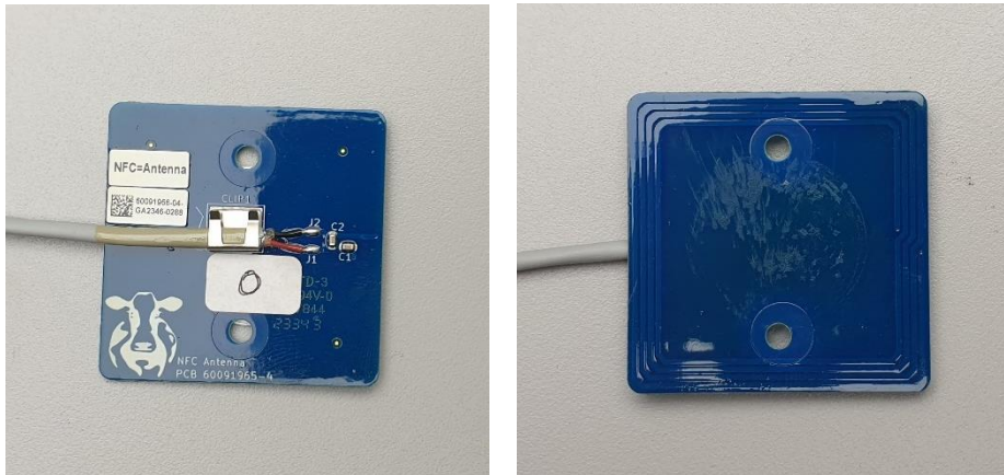
Photo 3. NFC Antenna. Without NFC Tag.
